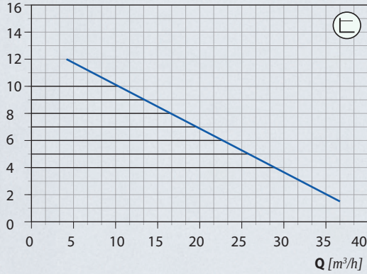
Sabit Basınç Değişken Debi Modu Fixed Pressure Variable Flow Mode
